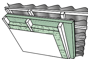
Aufsparrendämmung mit Zwischensparrendämmung
